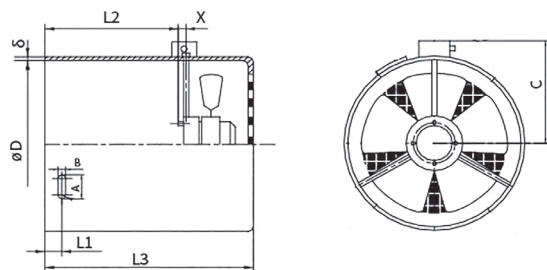
УНВ габаритные размеры тип В
